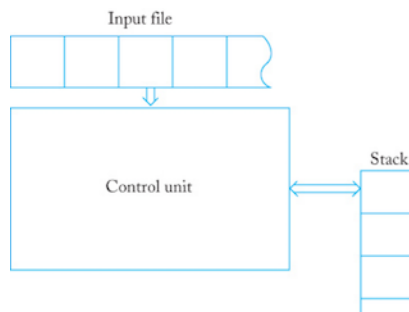
Linz Fig. 7.1: Pushdown Automaton
